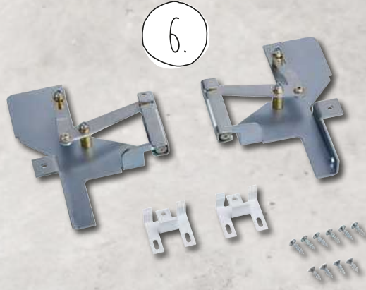
KLAPPSCHARNIER FÜR HOHE KORPUSMASSE Best.-Nr. Z 7880 X0
